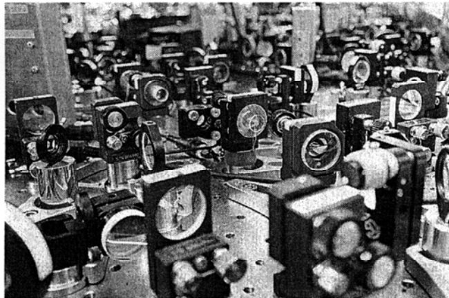
レンズや鏡が並ぶ「量子テレポーション」の実験装置（東京大の古沢明教授提供）
